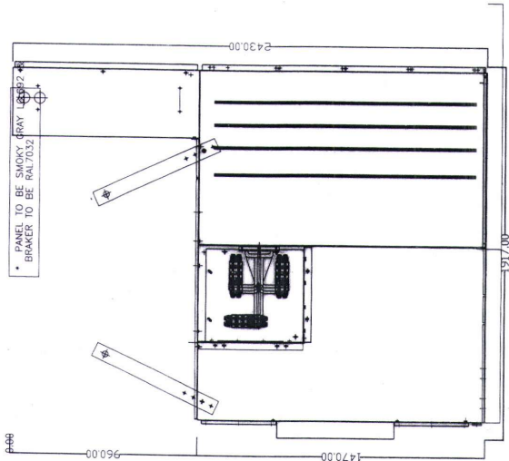
MOTOR FDR-1
